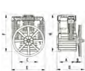
Σχεδιαγράμματα διαστάσεων K25, K28, K30 και K50
