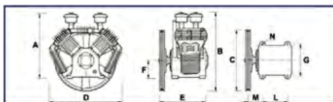
Διβάθμιες κεφαλές
